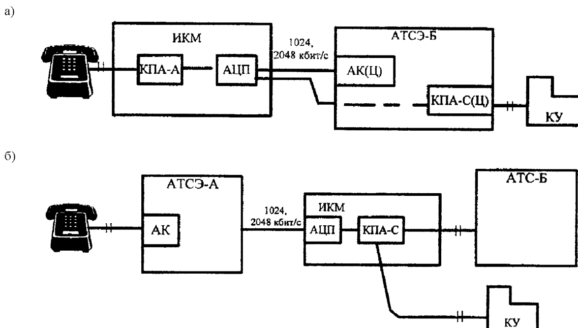
Рисунок 6.6. Реализации на АТСЭ абонентского (КПА-А) и станционного (КПА-С) окончаний для подключений прямого абонента
